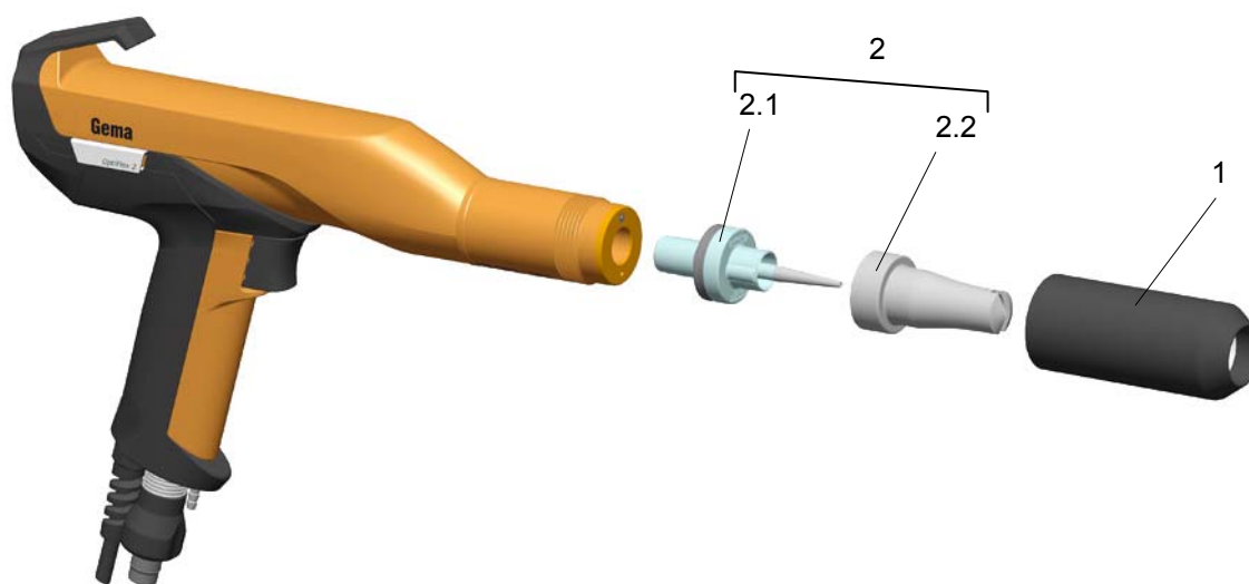
Ручной пистолет OptiSelect GM03 - Список запасных частей
